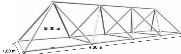
Χωροδικτύωμα
